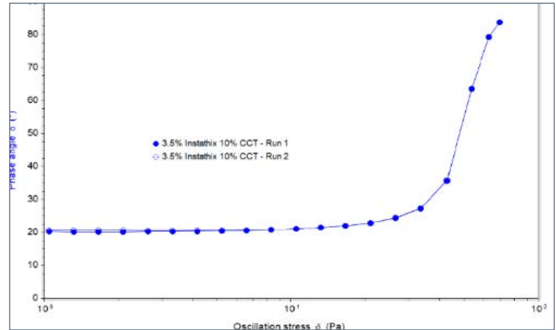
Фазовый угол (°) (мера упругости) в зависимости от колебательного напряжения (Pa)
